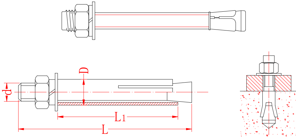
安装示意图
