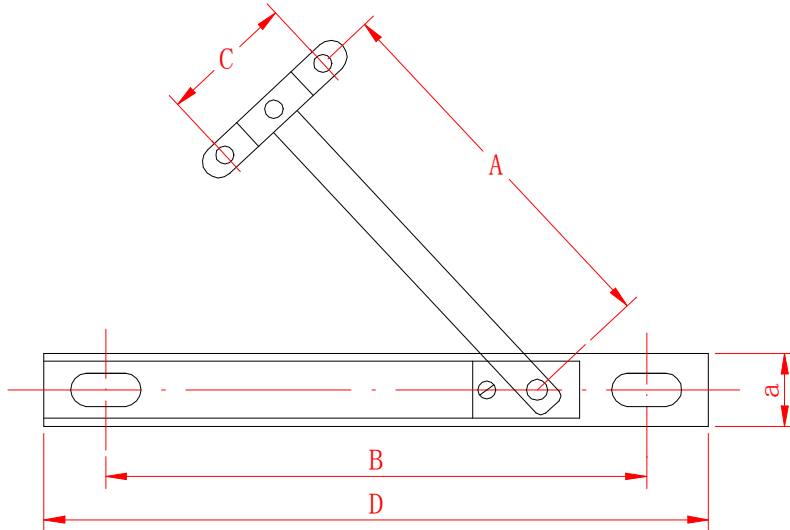
图6-1-3 幕墙窗撑
