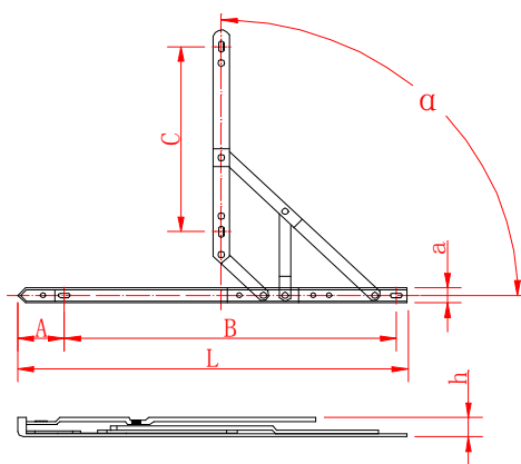
图6-1-1 (a) 平级型
