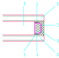
图 2.34 中空玻璃构造示意图
