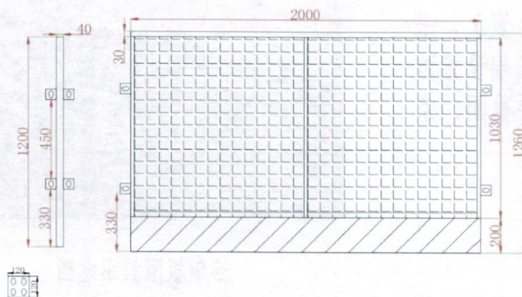
网片式围挡示意图
